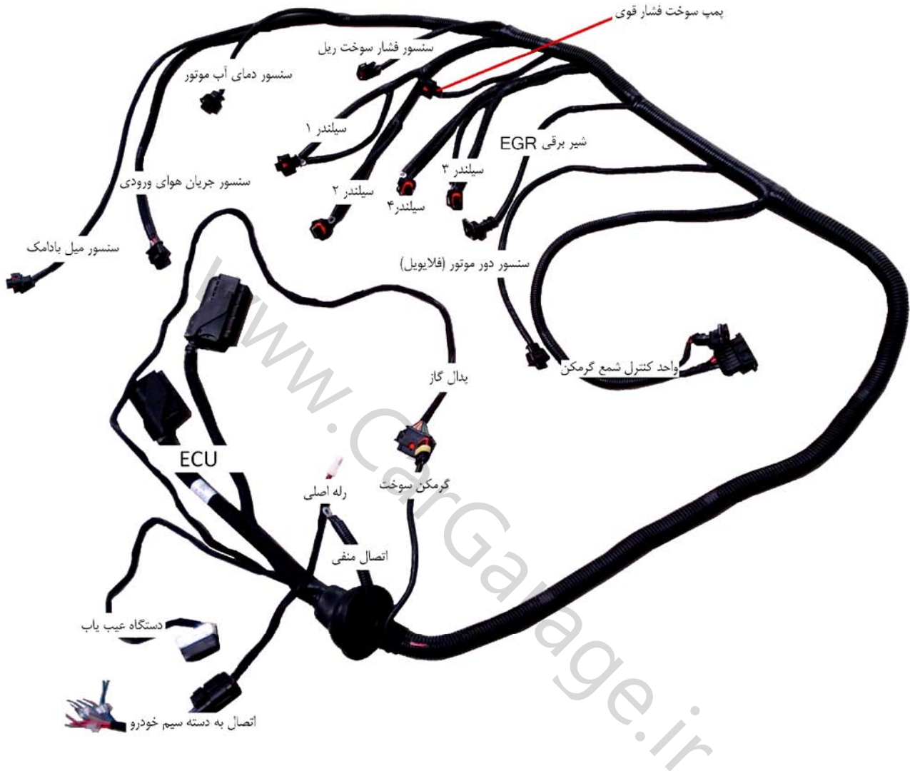
شکل ۴-۴: کابل اتصال موتور
